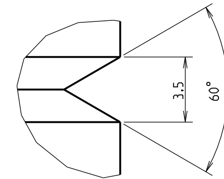
DETAIL A MASSSTAB 5:1
